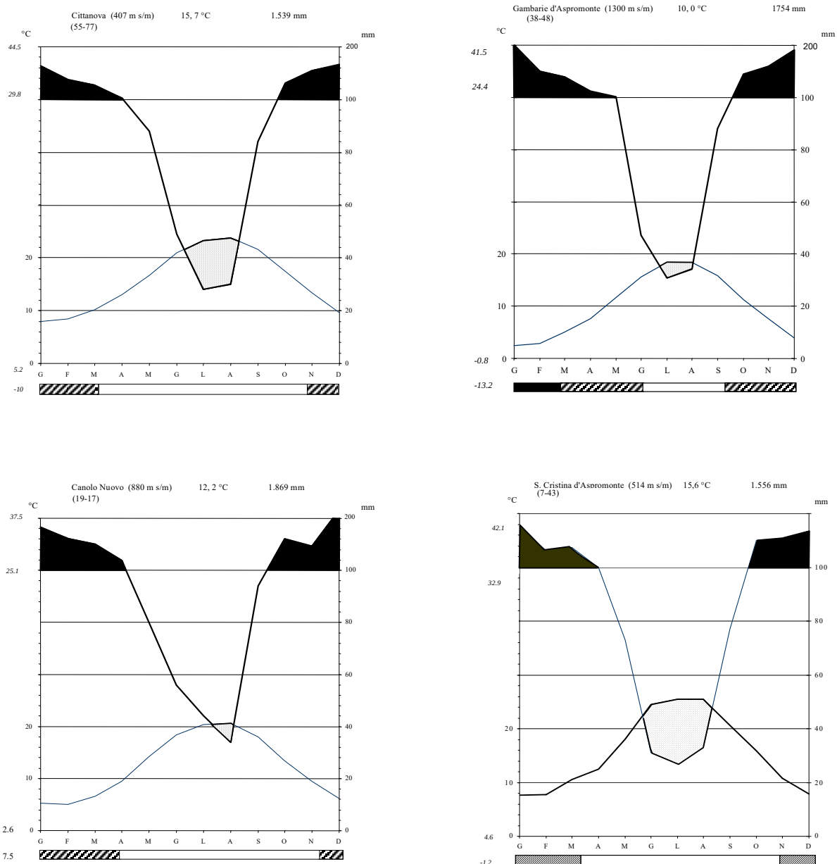
Figura 10 – Diagrammi ombrotermici.
